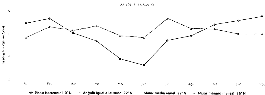
Irradiação Solar no Plano Inclinado - Monte Siao-Monte Siao, MG-BRASIL
